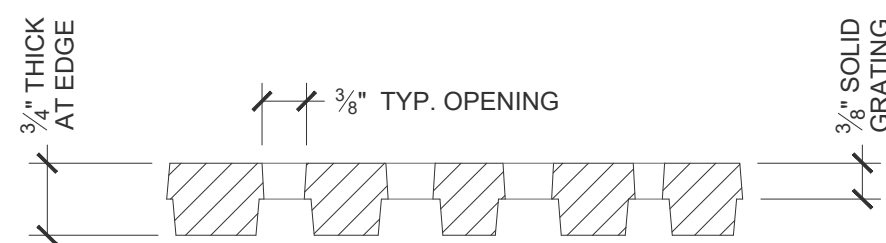
Cross Section Scale: 6" = 1' 0"
