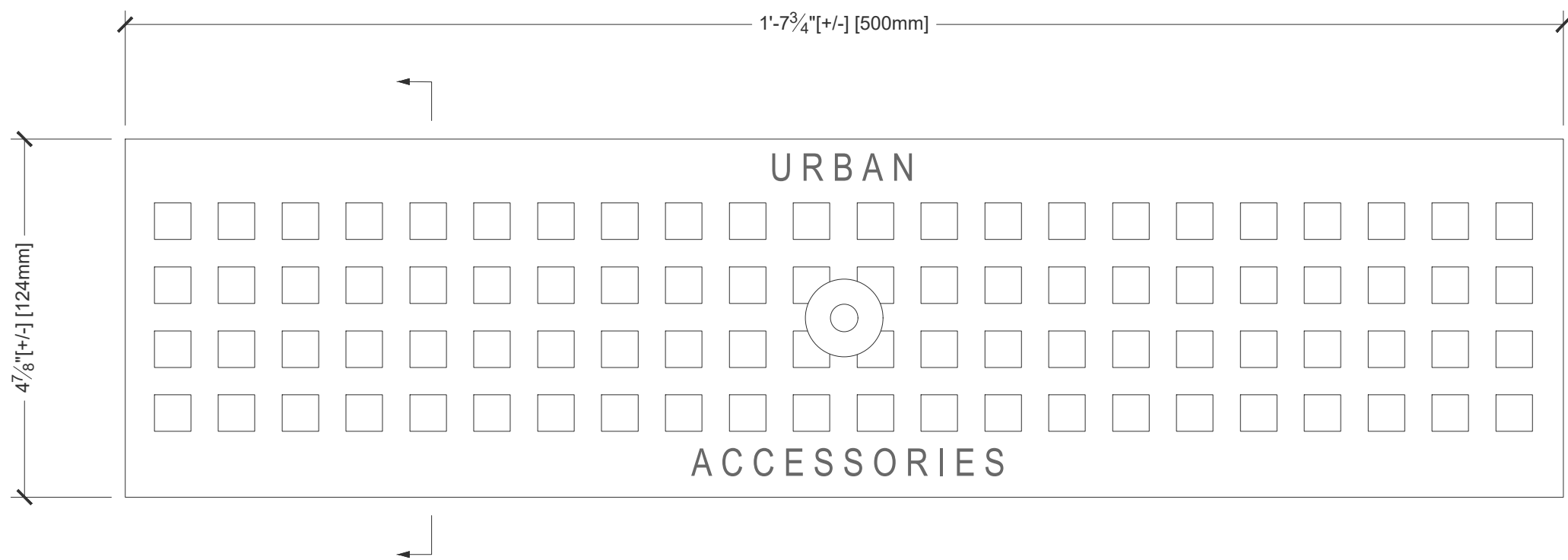
Plan Scale: 6" = 1' 0"
