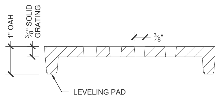
Cross Section Scale: 6" = 1' 0"
