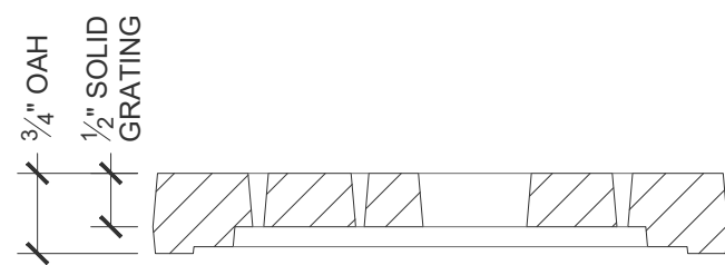
Cross Section Scale: 6" = 1' 0"
