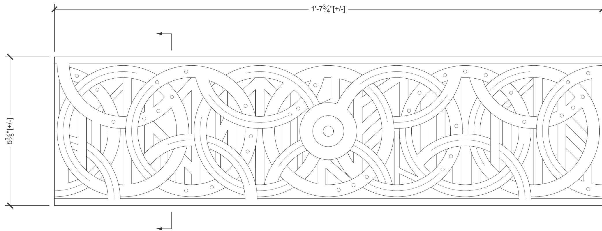
Plan Scale: 6" = 1' 0"
