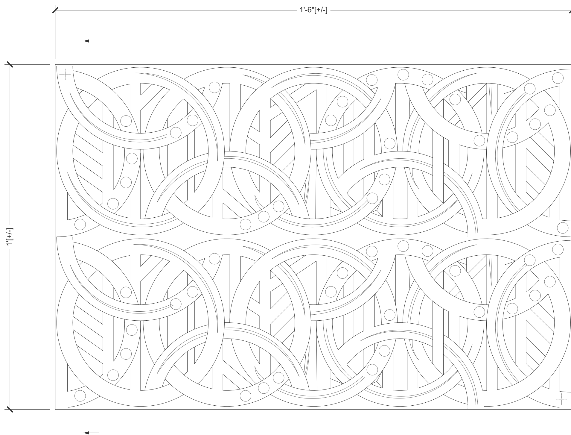
Plan Scale: 6" = 1' 0"
