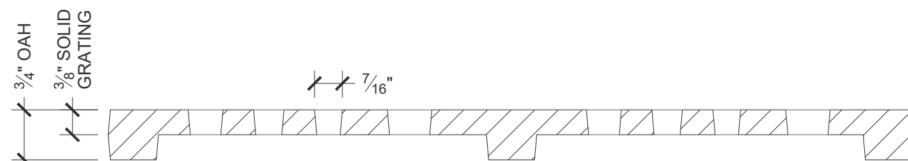
Cross Section Scale: 6" = 1' 0"
