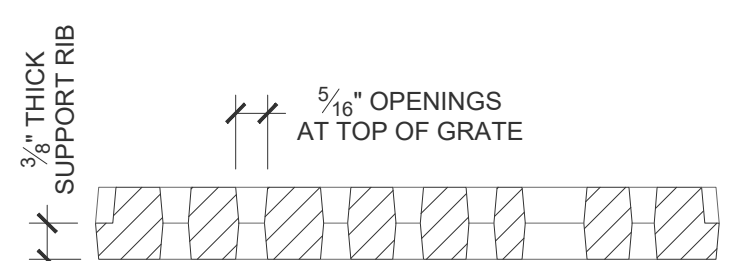
Cross Section Scale: 6" = 1' 0"
