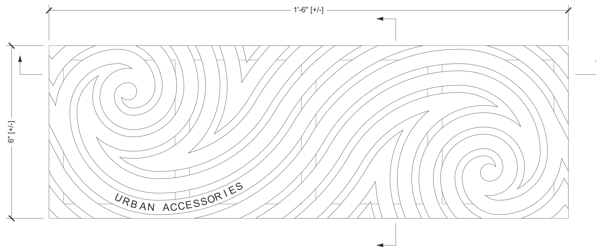
Plan Scale: 6" = 1' 0"
