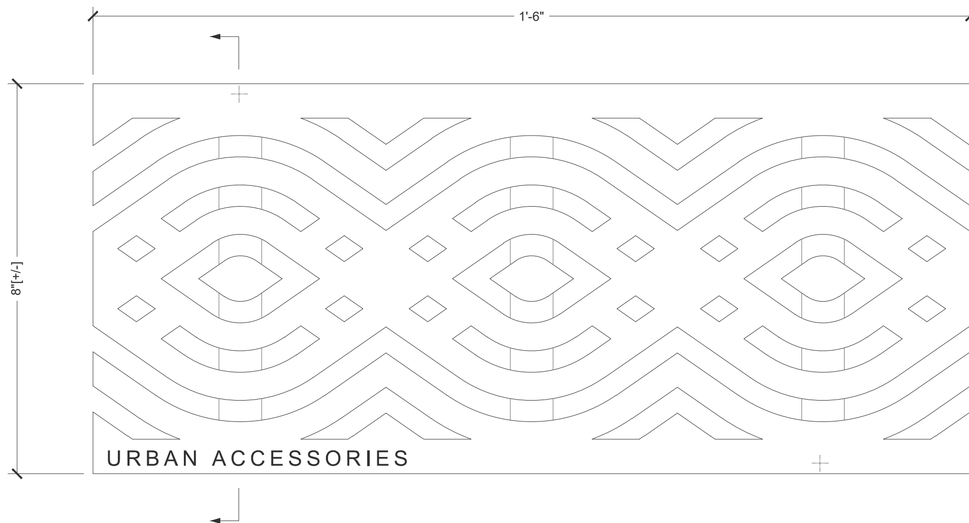
Plan Scale: 6" = 1' 0"
