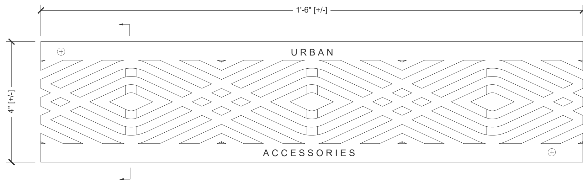
Plan Scale: 6" = 1' 0"
