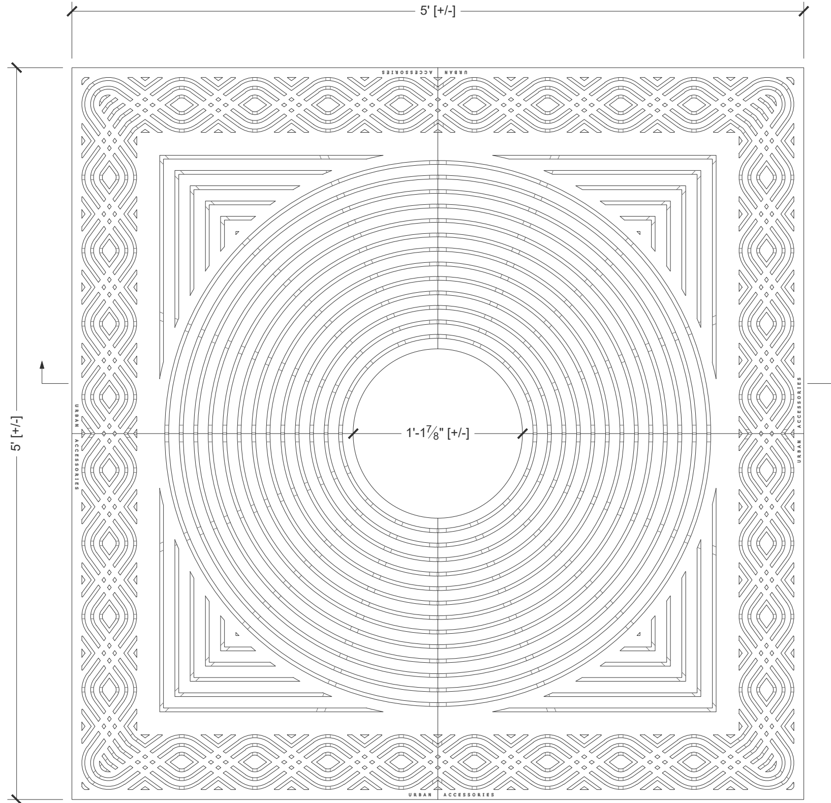
Plan Scale: 1 1/2" = 1' 0"
