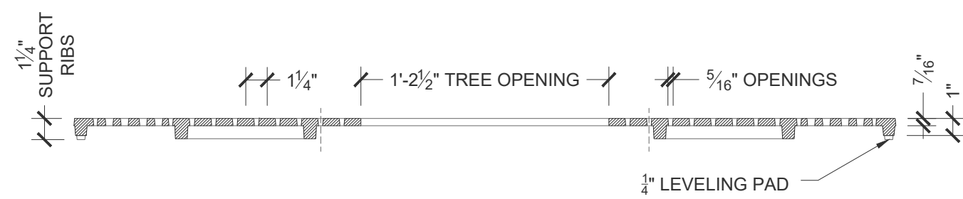
Longitudinal Section
