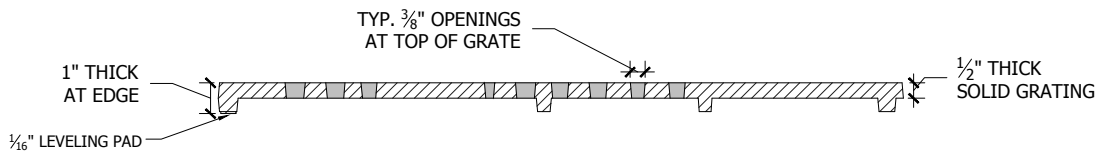
Section A-A'
