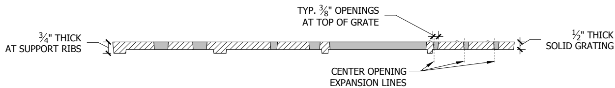
Section A-A'
