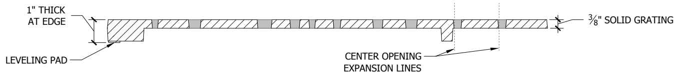
Section A-A'
