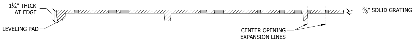
Section A-A'
