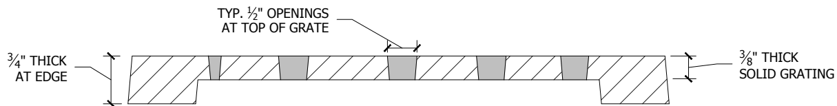
Section A-A'
