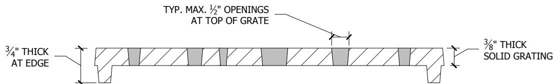
Section A-A'
