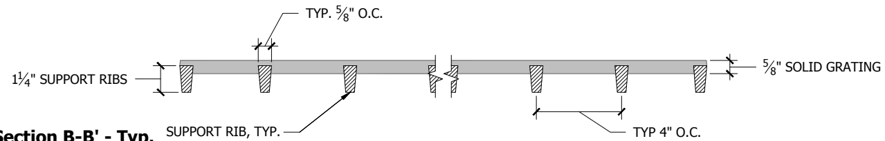
Section B-B' - Typ.
