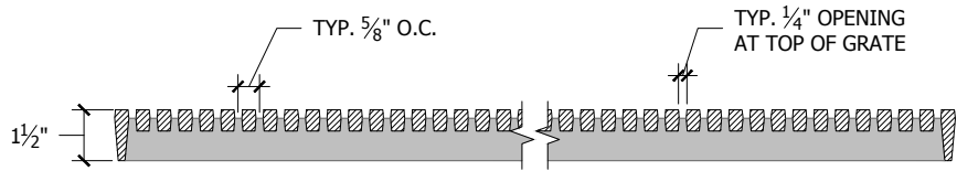
Section A-A' - Typ.
